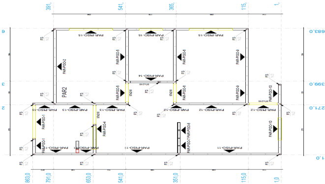
Planta de modulação do pavimento PISO - Fada 01
