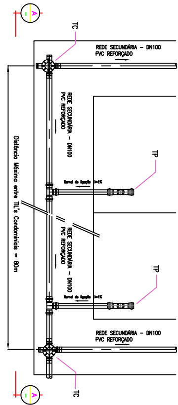
DETALHE LIGAÇÃO – S/ESC
